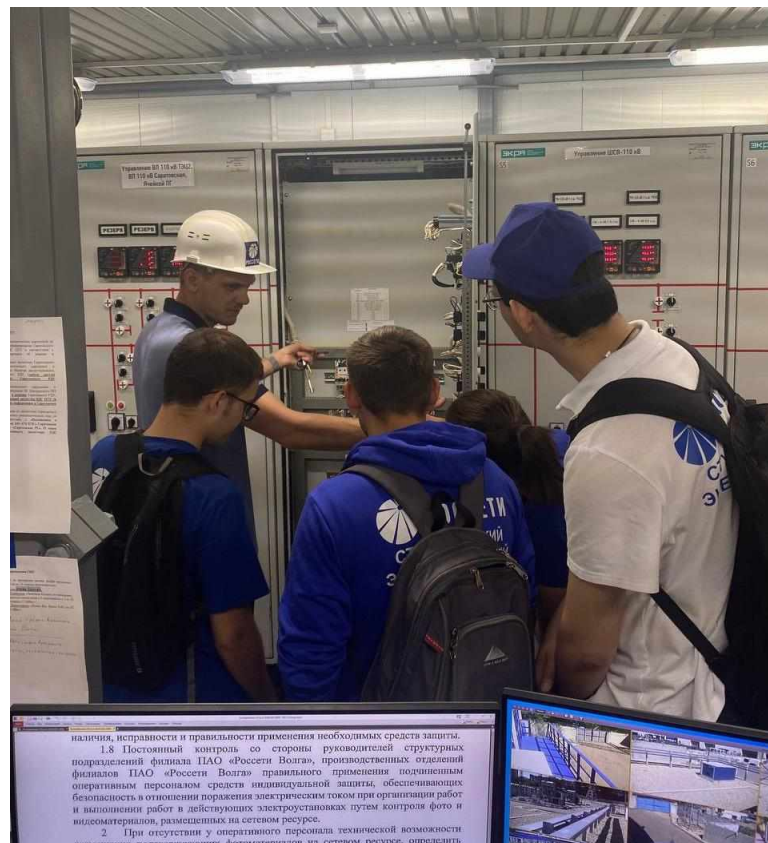
Рис.37. Отряд «Импульс». Проверка блокировок вводно-распределительного устройства.
